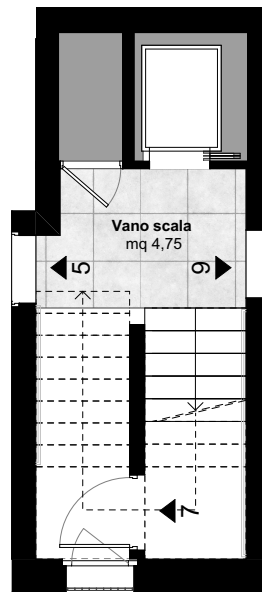
Piano Secondo (Scala 1:100)
